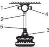
g.吊杆式
