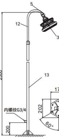
h: 法兰式
