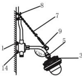
b2: 壁式30°
