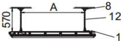
吊链式(L)
