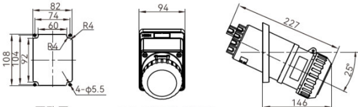
开孔图
