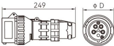
T-插头
