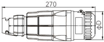
LZ-连接器插座
