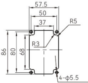
开孔图
