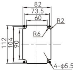
开孔图
