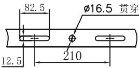
I型 安装孔位
