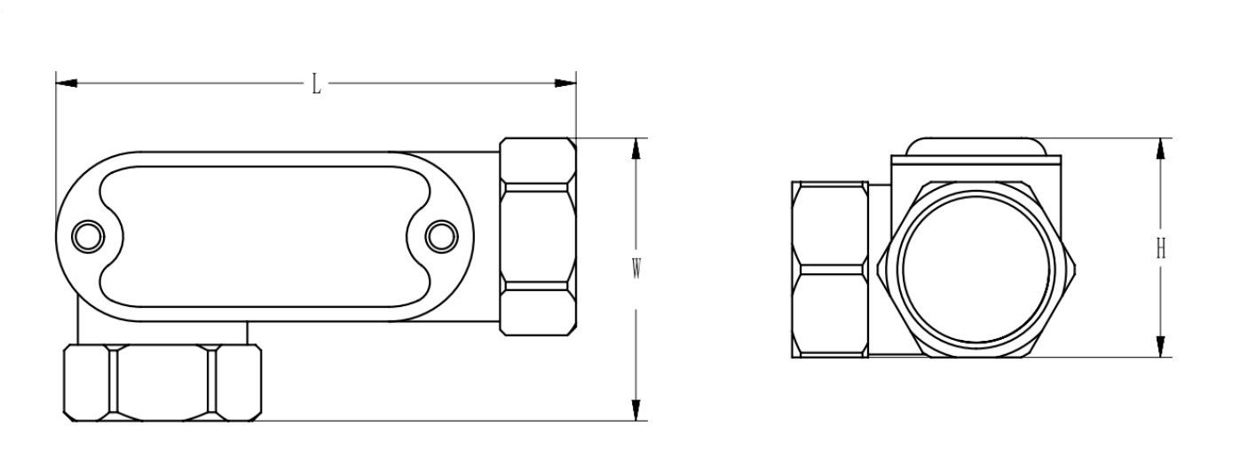
SZ-BHC不锈钢E型H/L/W配套图
