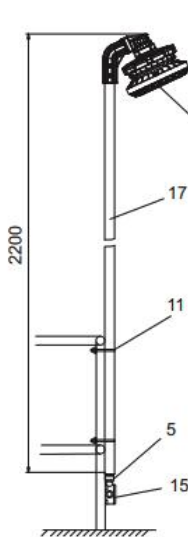
f: 护栏式
