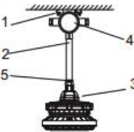
g.吊杆式
