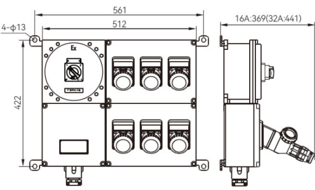
配16(32)A插销示意图
