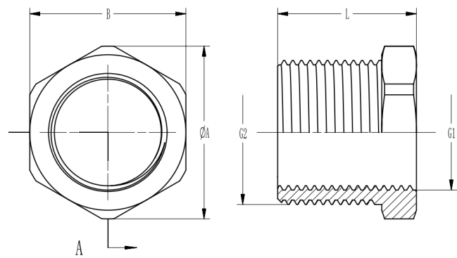
外形尺寸代号图
