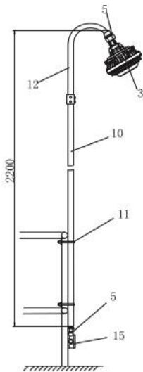
f: 护栏式
