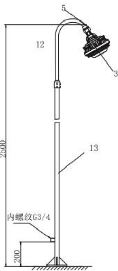
h: 法兰式
